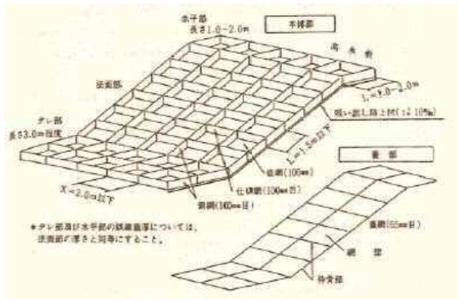
図 1-4 護岸構造（低水護岸：根固め工がない場合）
