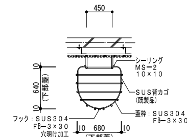
底部平面图
