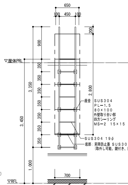
H3350 正面図
