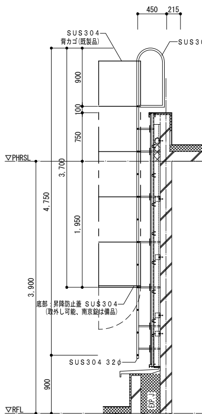
H4750 側面図
