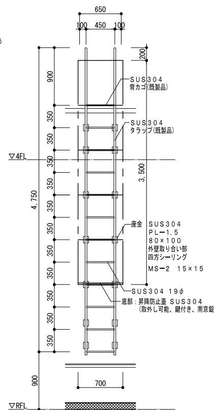
※3F~4F H4750正面図
