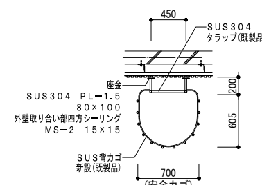
上部平面图
