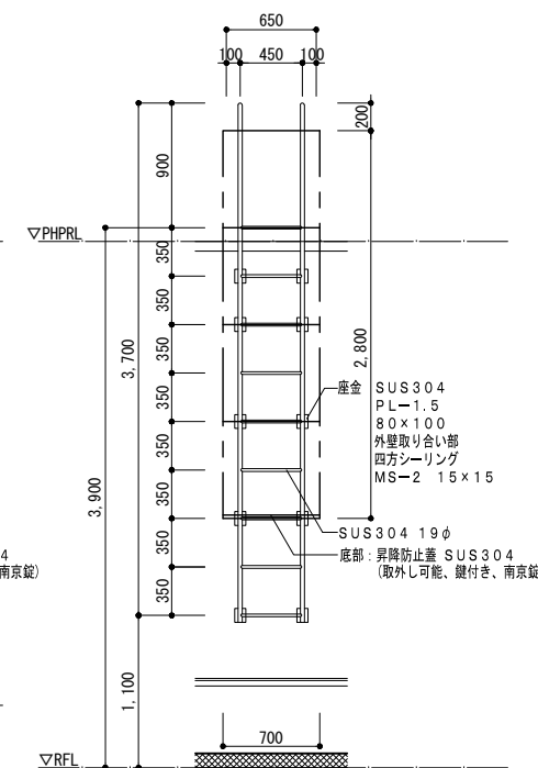
H3700 正面図
