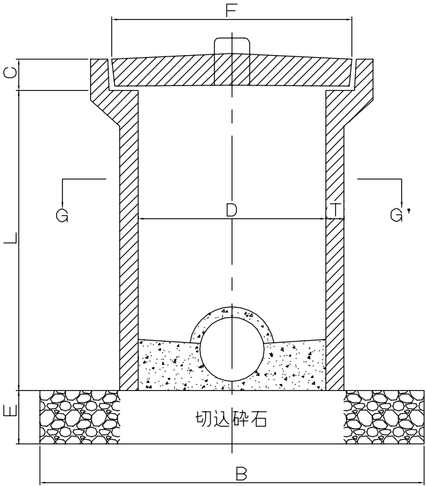
縦断面図
