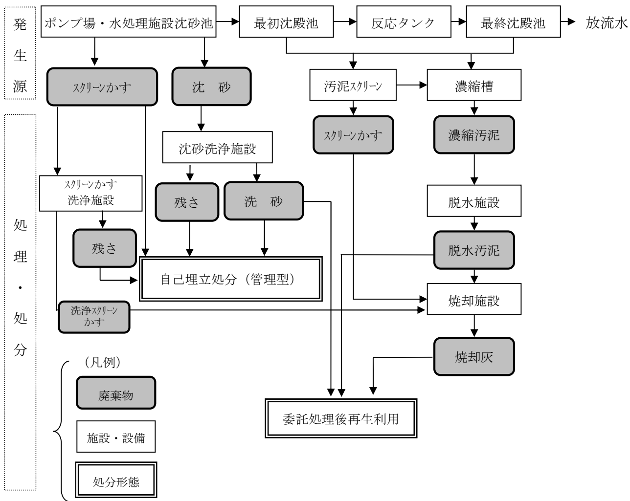
図1 処理フロー
