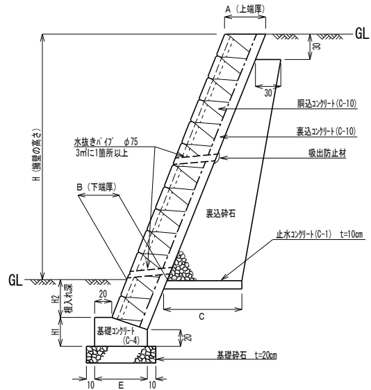
練積み擁壁断面図 1/〇〇
