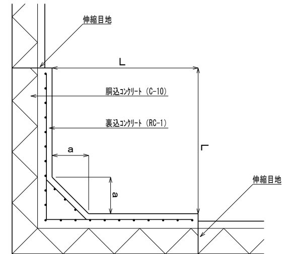
隅角部詳細図 1/〇〇
