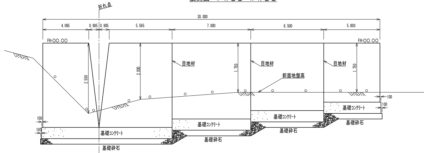
展開図 V=1/〇〇 H=1/〇〇
