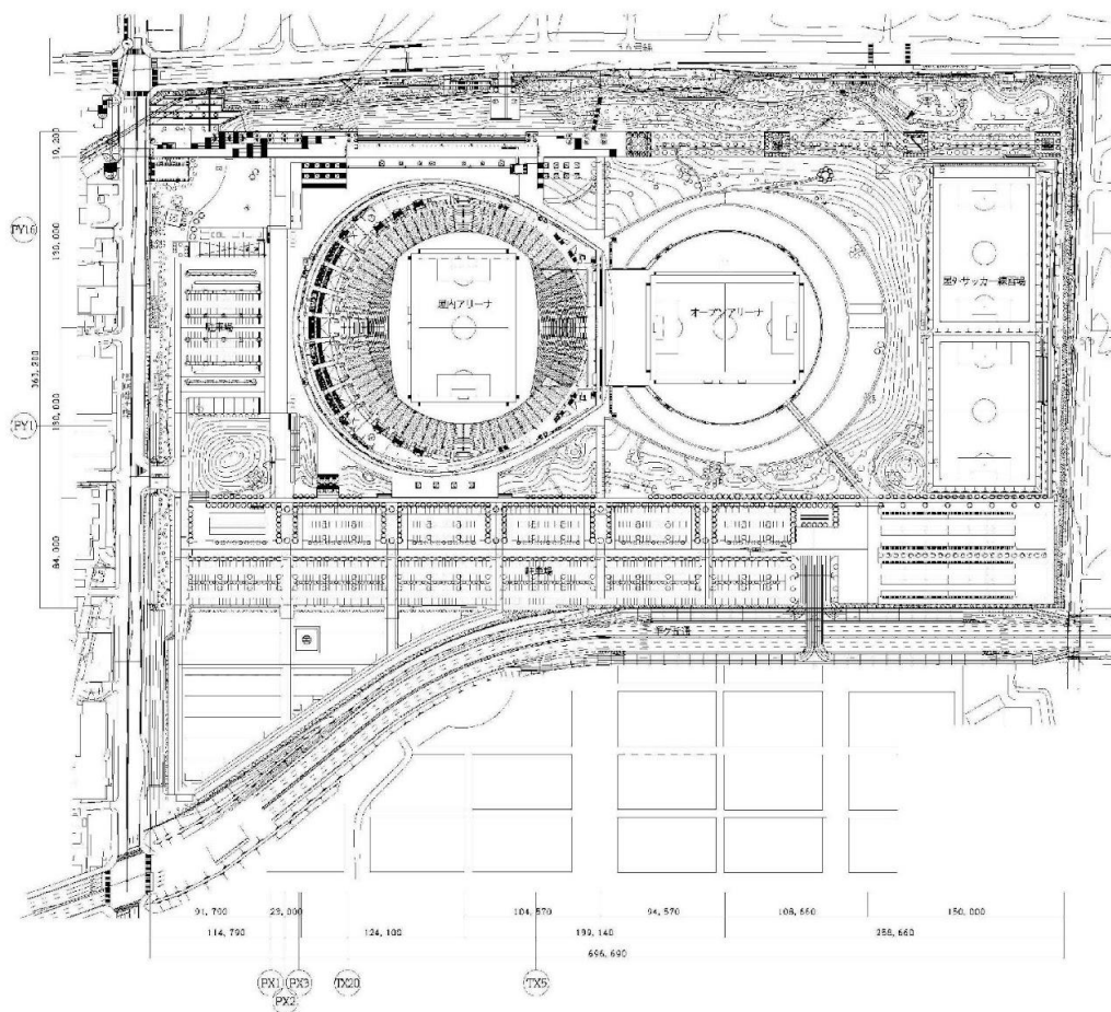
配置図
