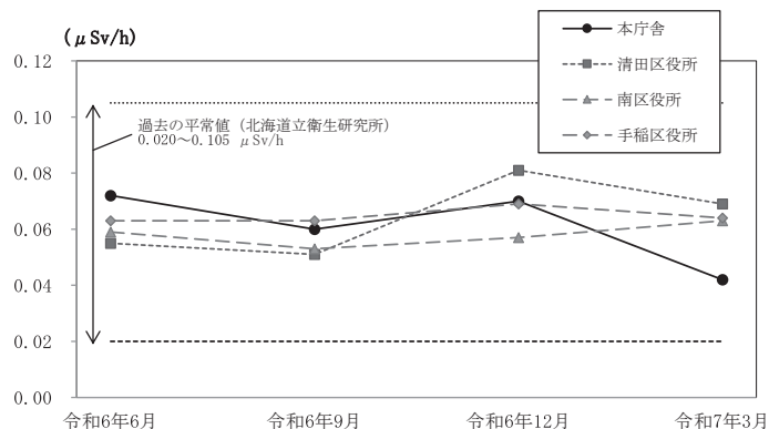
図2-1-9 環境放射線量(令和6年度)
