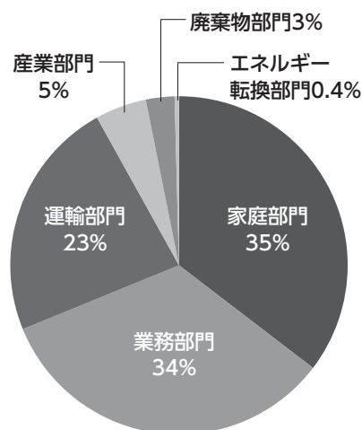
図2-2-2 札幌市における二酸化炭素排出量の部門別内訳
