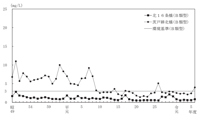
図 2-1-12 BODの経年変化(茨戸川水域 環境基準点)
