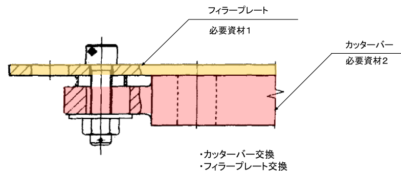
カッターバー取付図
