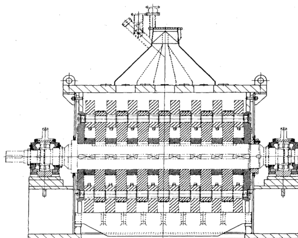
断面 A-A
