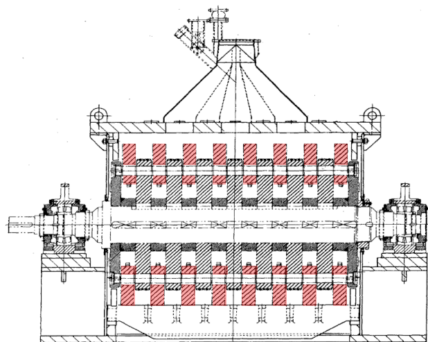
断面A-A
