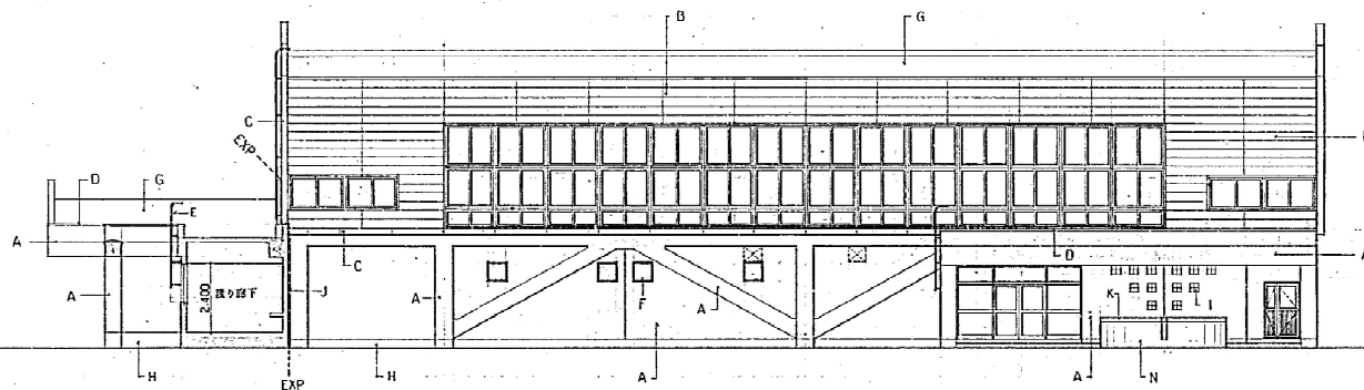
西立面図 1:100
