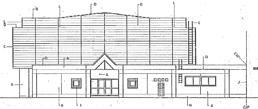
北立面図 1:100
