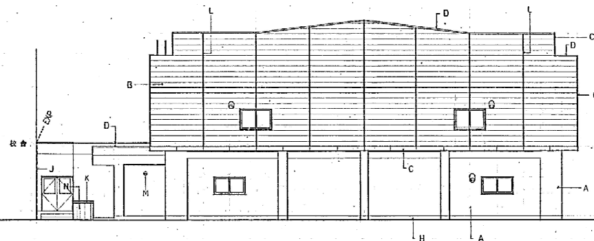
南立面図 1:100
