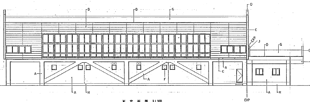
東立面図 1:100
