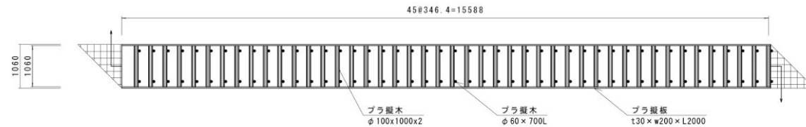
展開図 S=1/40
