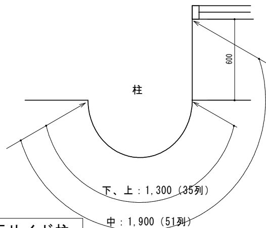
両サイド柱
