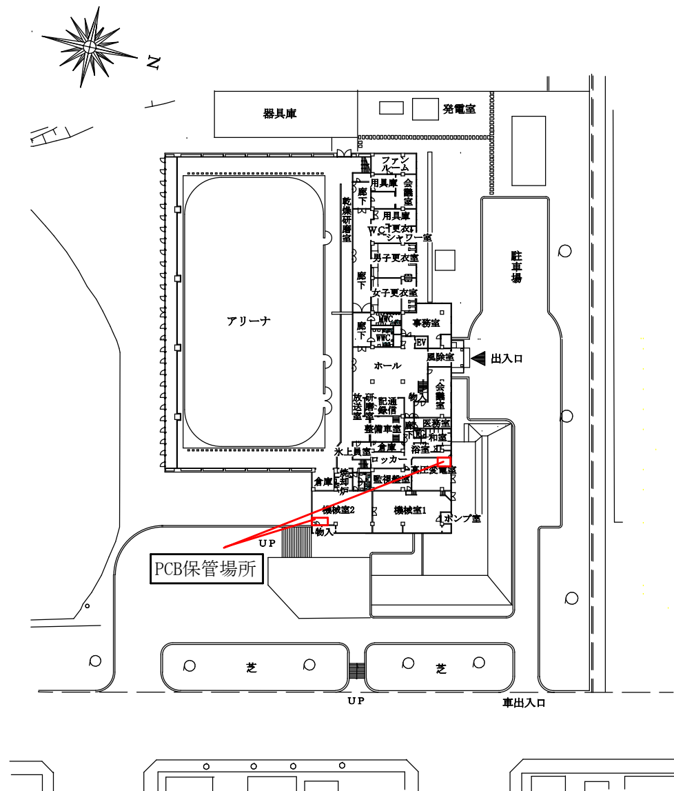
配置図
