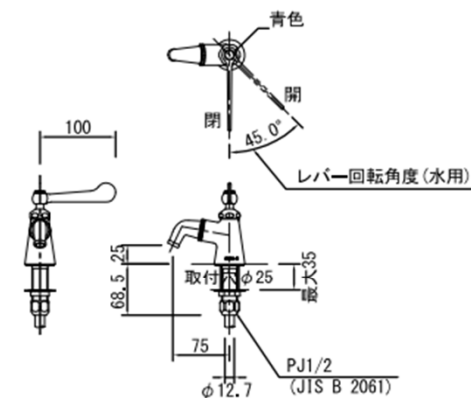
手洗い水栓詳細図 S=1/10
