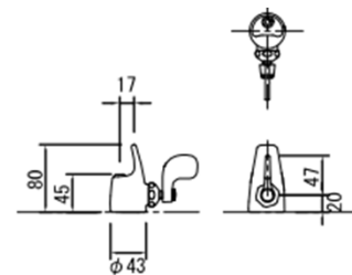
水飲み水栓詳細図 S=1/10
