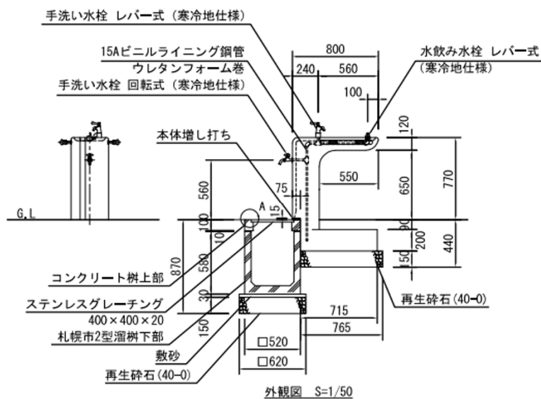
外観図 S=1/50
