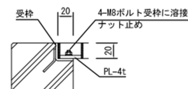
A部詳細図 S=1/5
