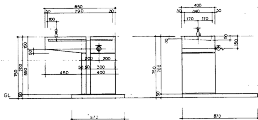
立面図
