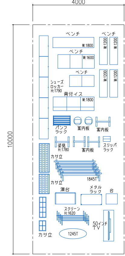
■ 2.3 F-下足スペース、廊下階段室2
