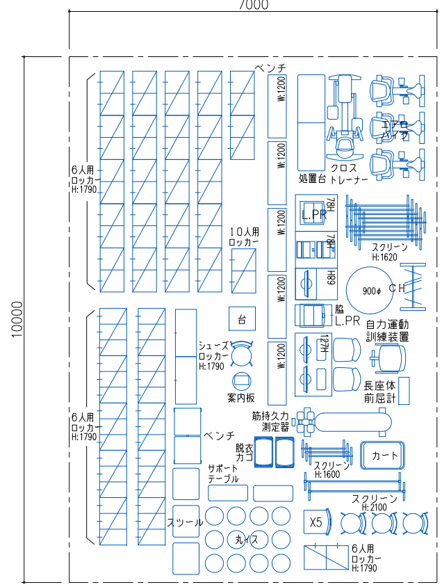
■ 2 F-更衣室、体力測定室
