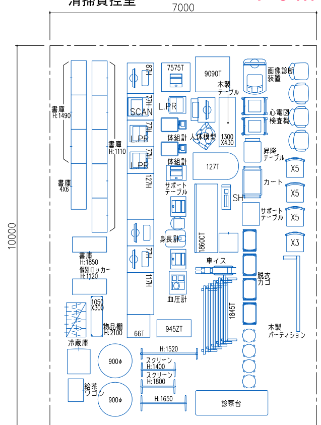
■ 3 F-研修室、栄養指導室、清掃員控室
