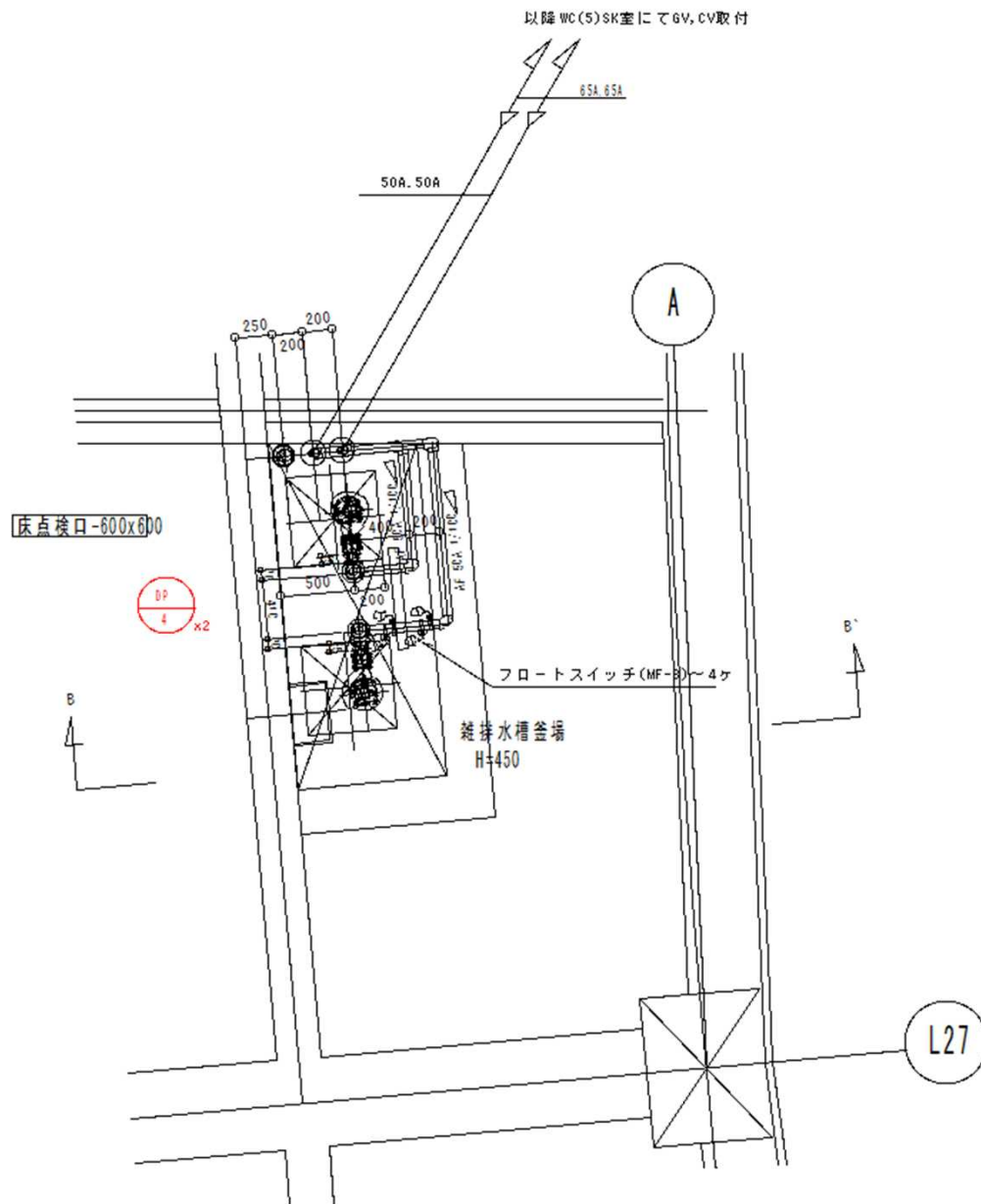
B2階平面図
