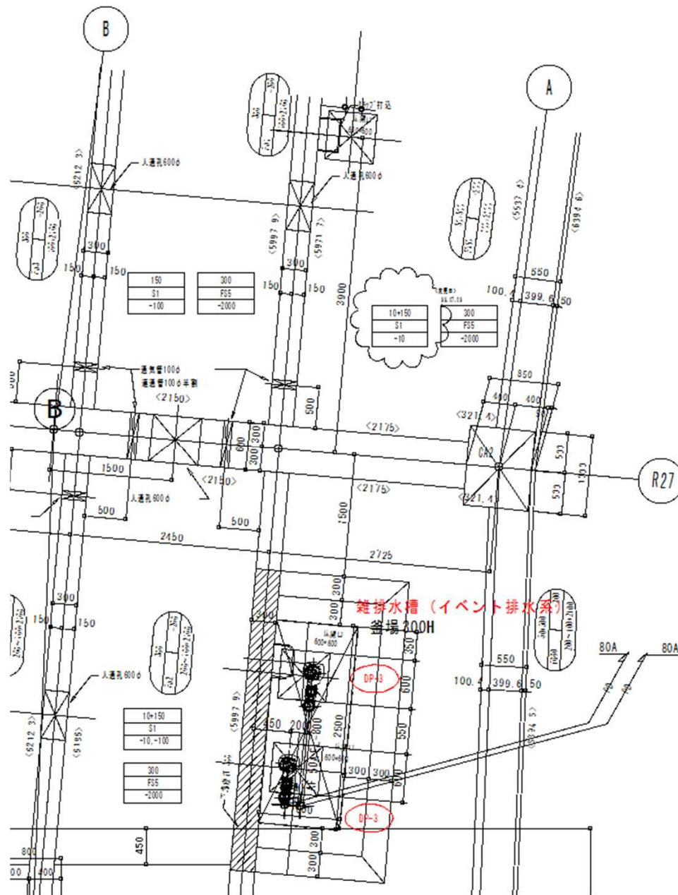
B2階平面図
