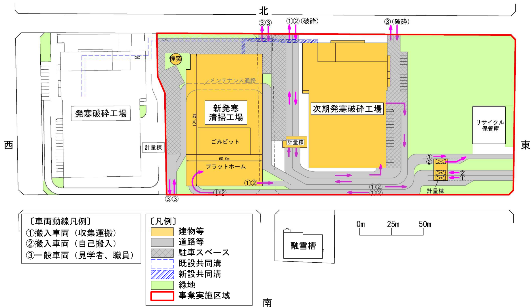
図 10.9 動線計画案（次期発寒破碎工場の建設時）
