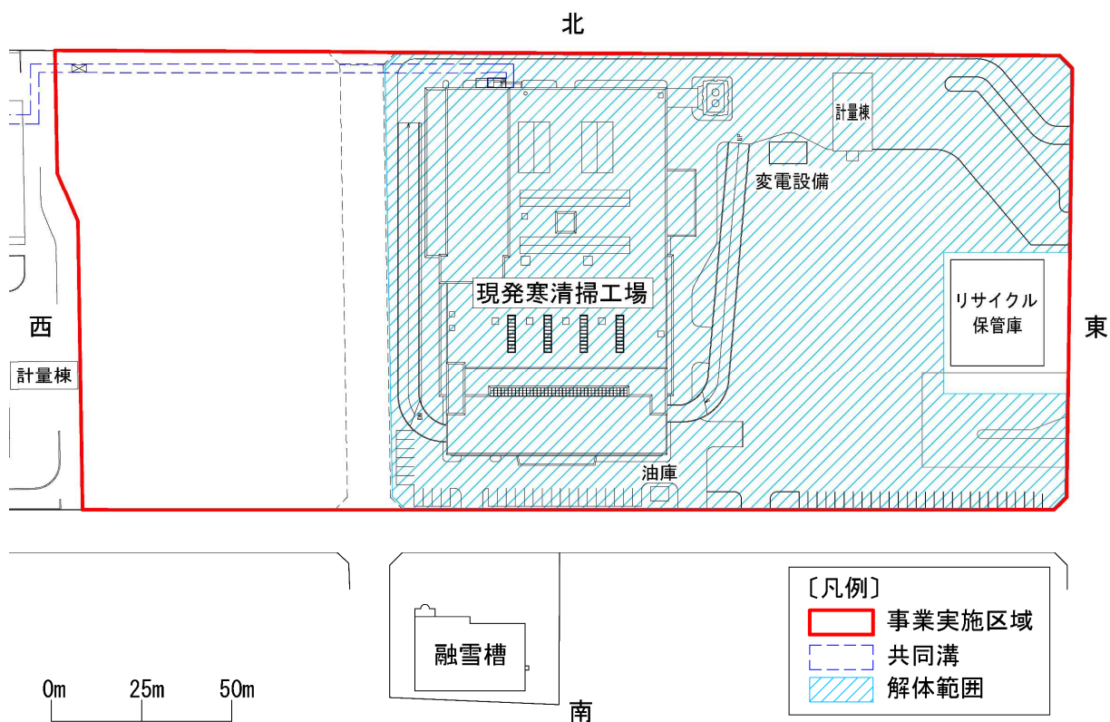
図 10.10 解体範囲
