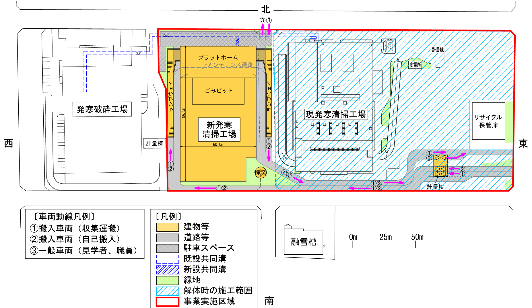
図 10.4 施設配置案（Aパターン：煙突南東側配置）
