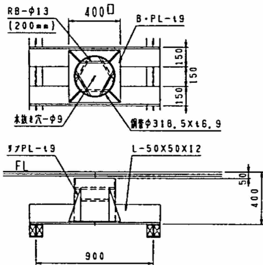
競技室 床金具詳細図（新築図面）
