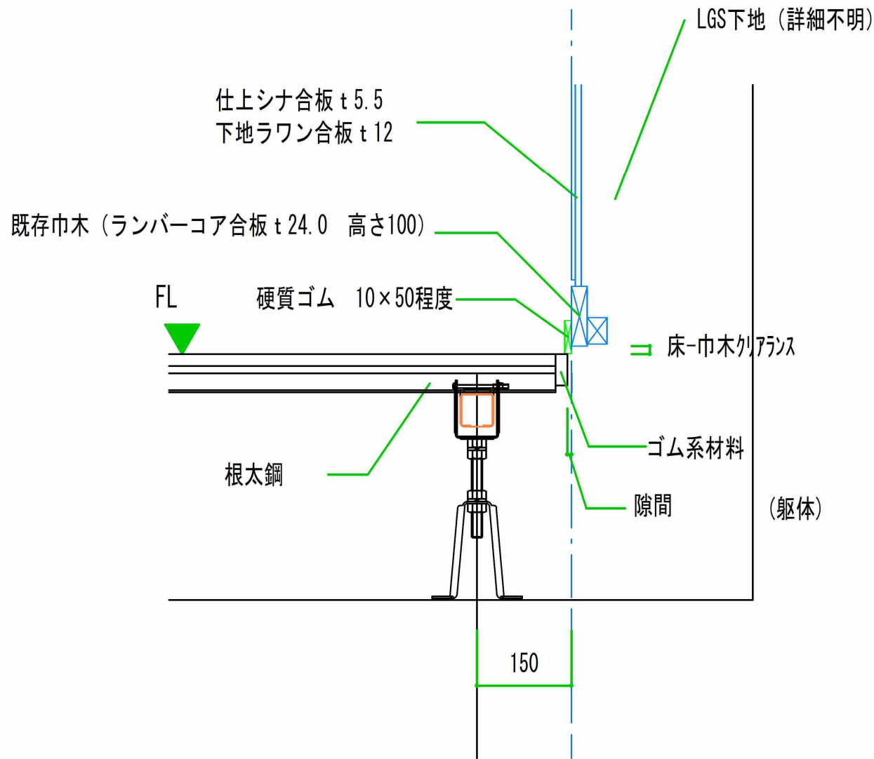
巾木部 硬質ゴム取付詳細図
