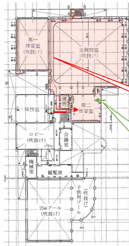
2階平面図
