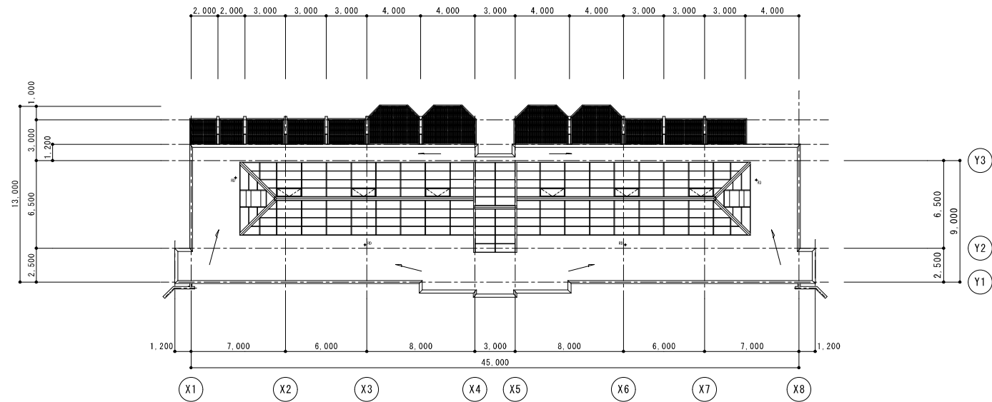
屋根伏図
