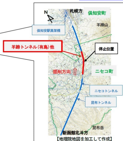
羊蹄トンネル(有島)他 延長= 4,245m
