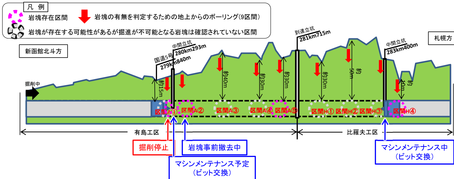
羊蹄トンネル(有島)他 延長= 4,245m
