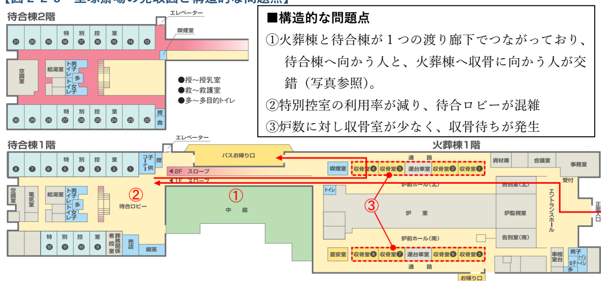
【図 2-2-5 里塚斎場の見取図と構造的な問題点】
