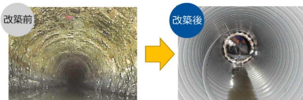
管更生工法による管路の改築
