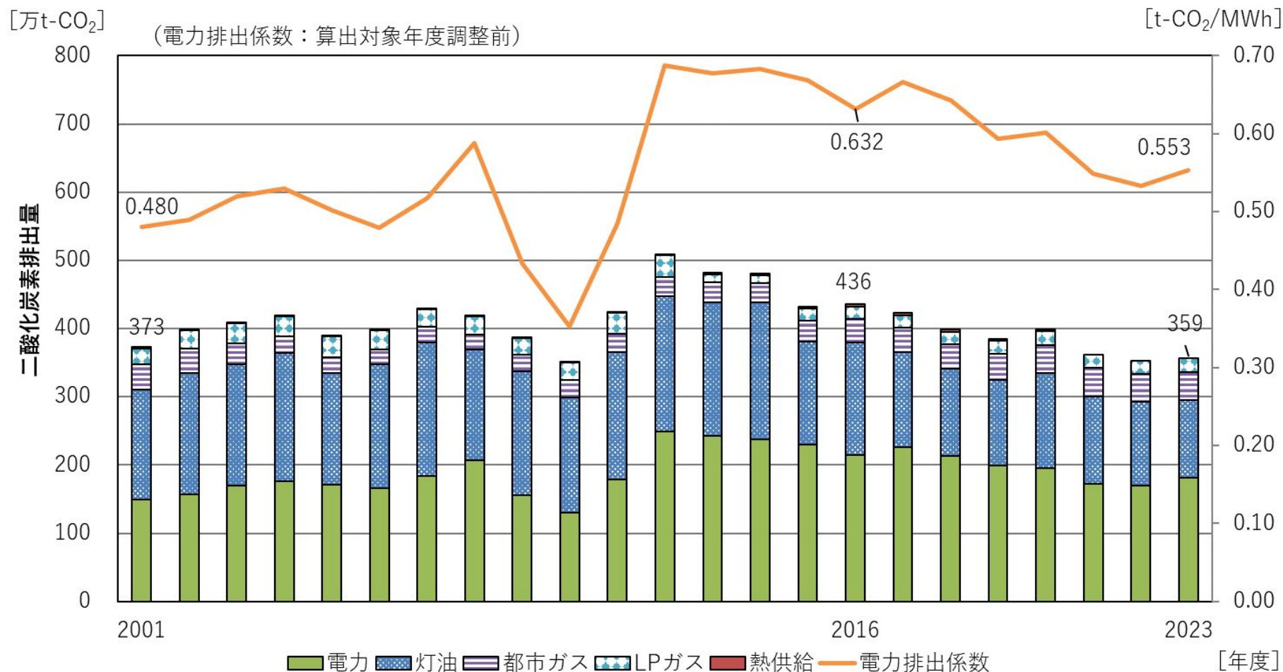
図 家庭部門の二酸化炭素排出量と電力排出係数の推移
