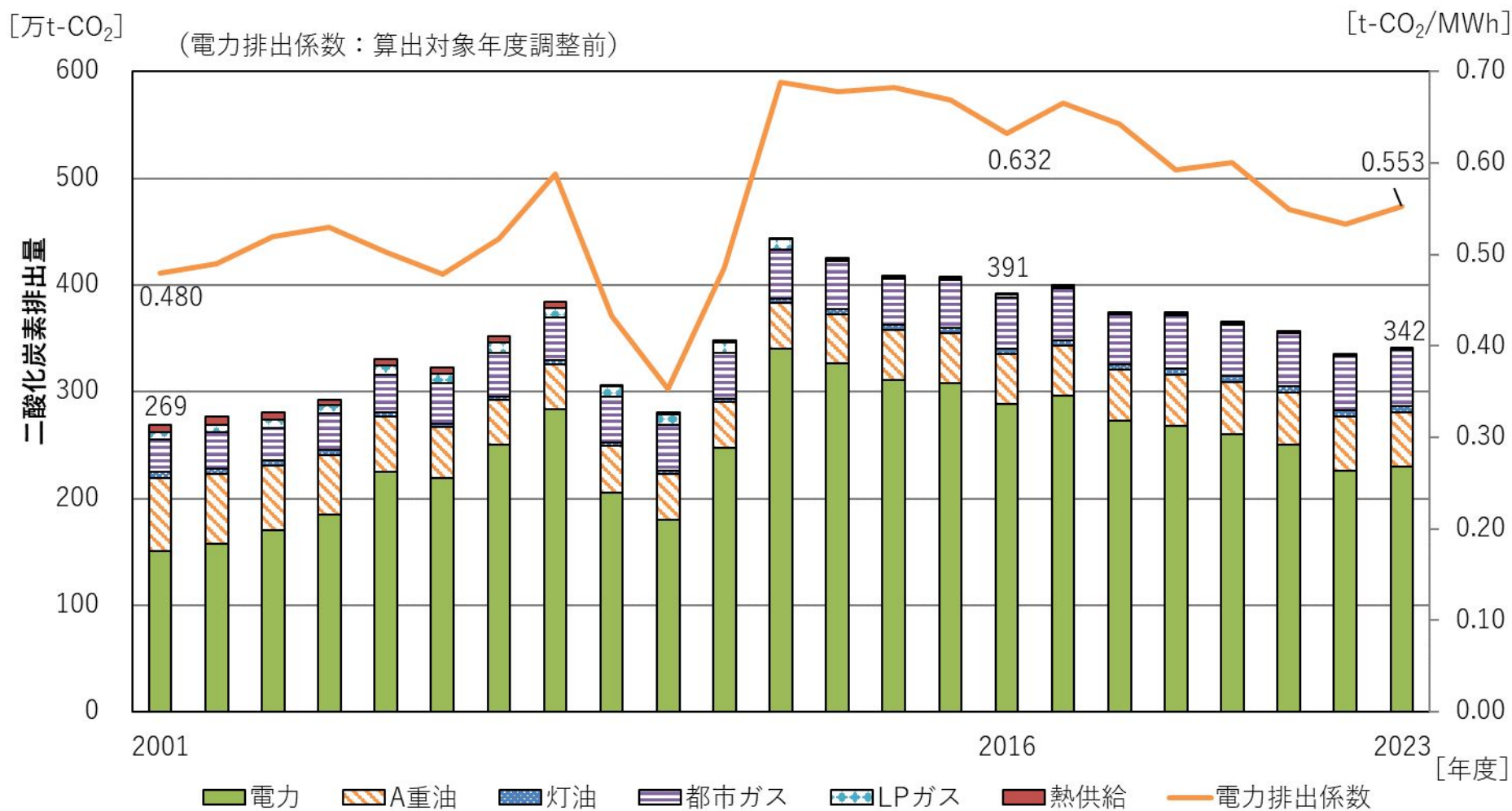
図 業務部門の二酸化炭素排出量と電力排出係数の推移
