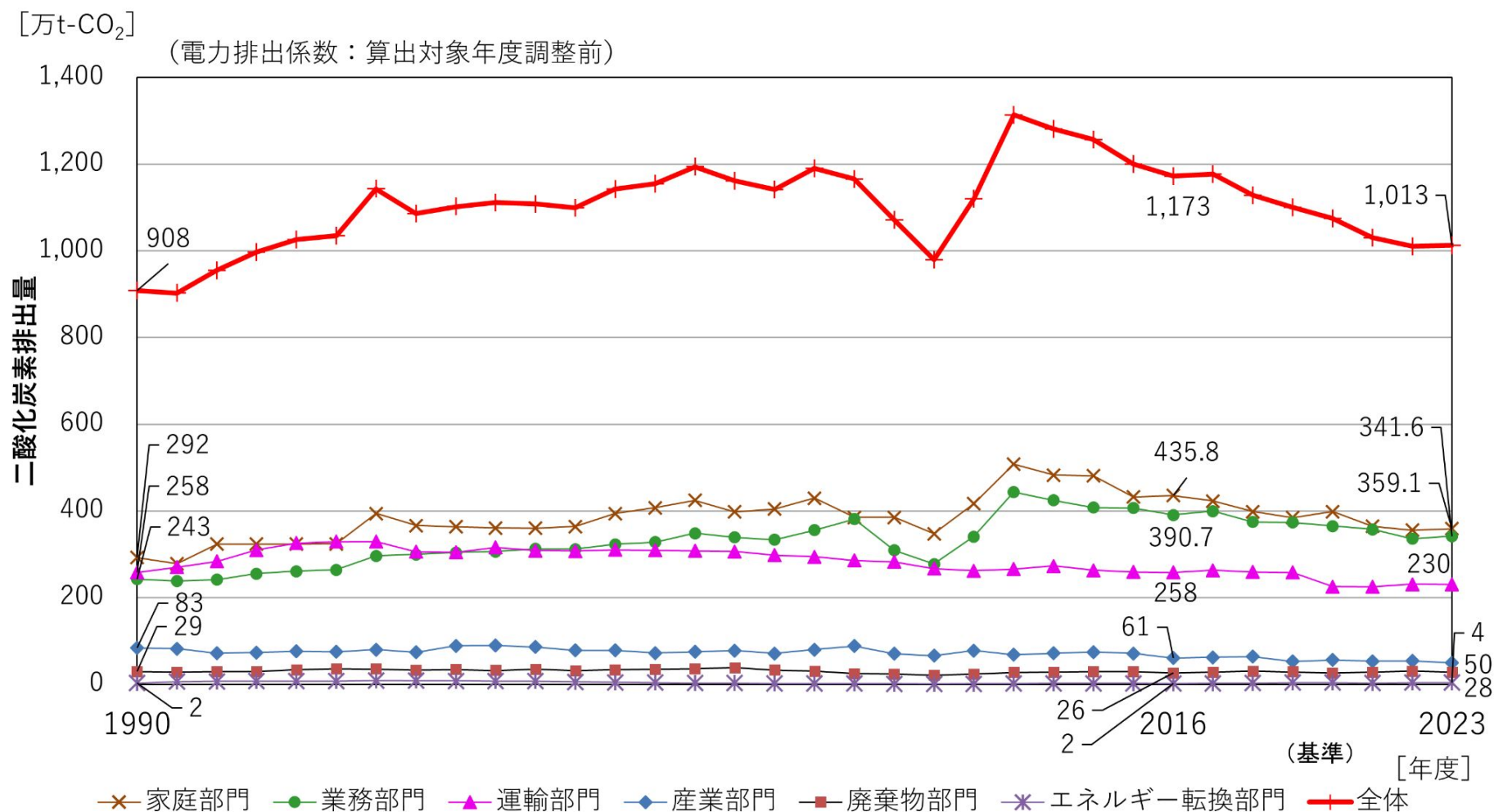
図 二酸化炭素排出量の部門別推移
