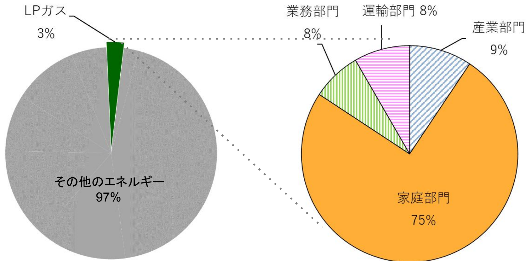
図 LPガス由来の二酸化炭素排出量の部門別内訳
