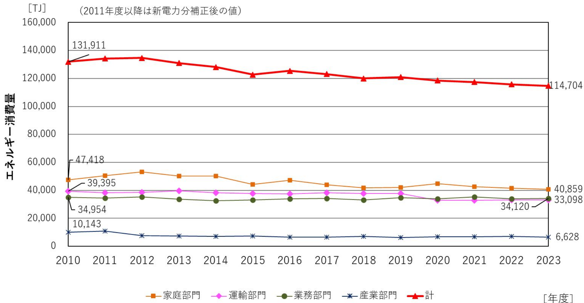
図 エネルギー消費量の部門別推移
